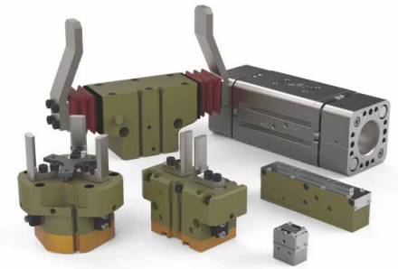
Parallelgreifer
