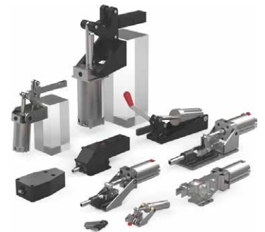
Pneumatische Standard-Kraftspanner
